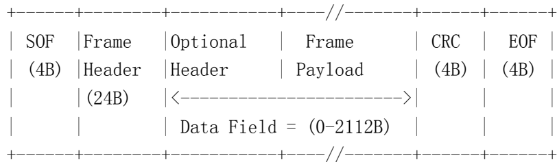
Fig. 16 FC Frame Format
