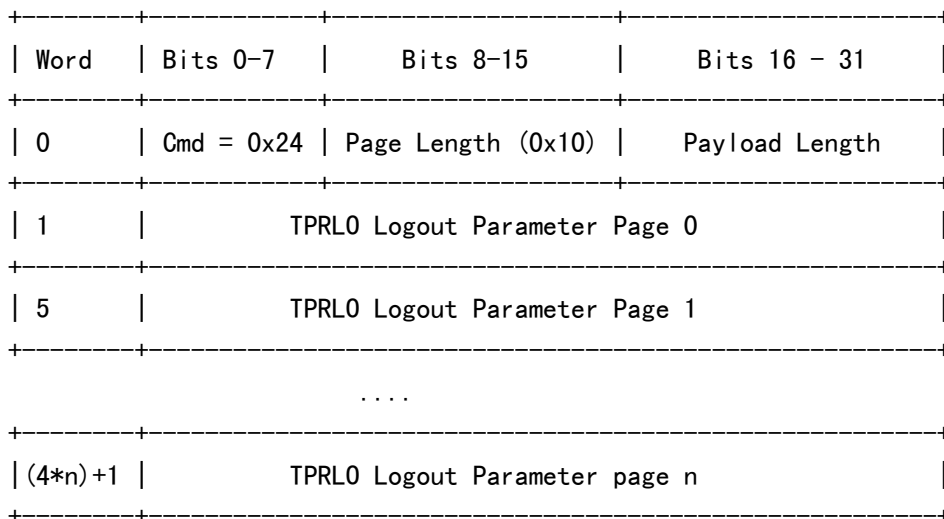
Figure 22 -- Format of TPRLO ELS
